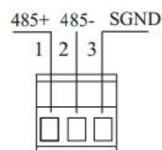
RS-485 output interface
